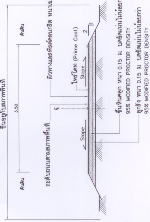
รูปตัด A
